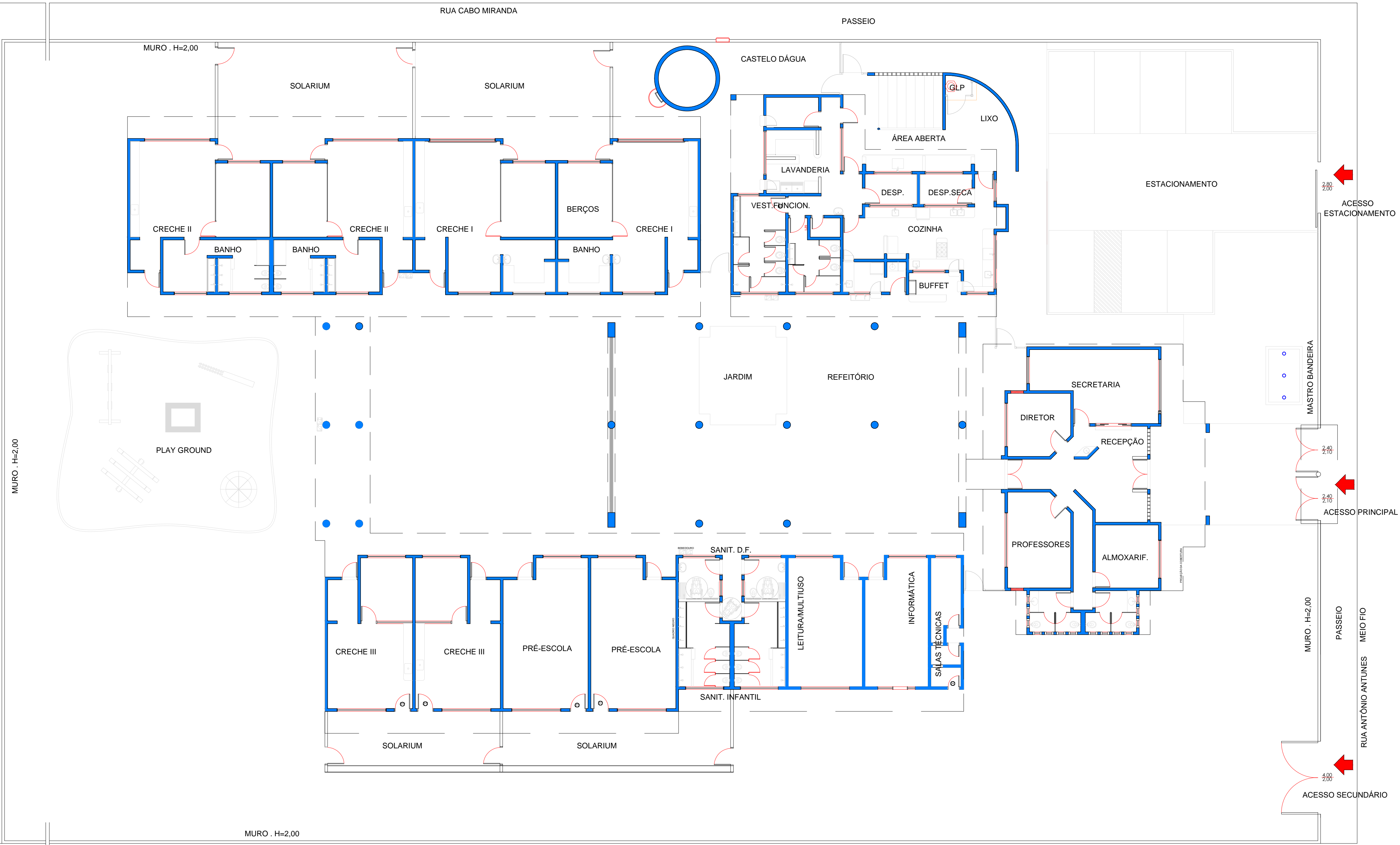
Planta de Implantação Escala 1:125
