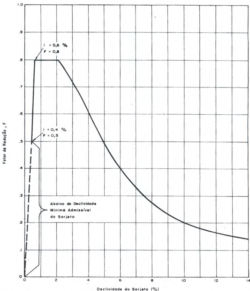
Gráfico 1. Fator de redução da capacidade de escoamento da sarjeta
