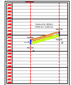
TRECHO J4 - J5 ESCALA - H= 1:250 V= 1:2500
