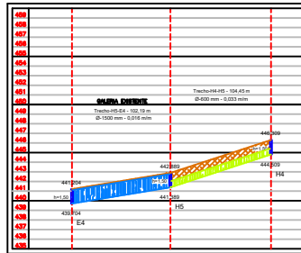
TRECHO H4 - E4 ESCALA - H= 1:250 V= 1:2500
