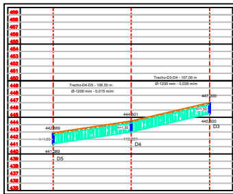
TRECHO D3 - D5 ESCALA - H= 1:250 V= 1:2500
