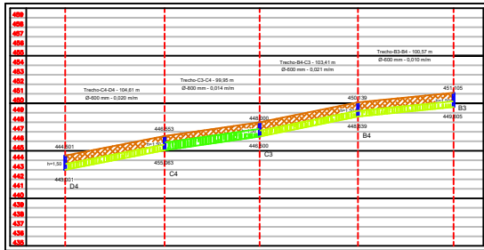
TRECHO B3 - D4 ESCALA - H= 1:250 V= 1:2500
