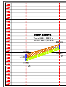
TRECHO I5 - E5 ESCALA - H= 1:250 V= 1:2500
