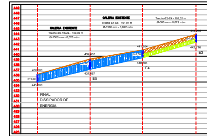
TRECHO E3 - FINAL ESCALA - H= 1:250 V= 1:2500
