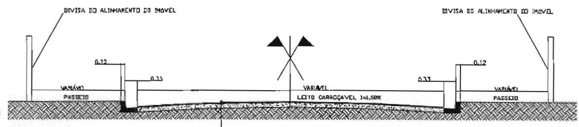
DETALHE DO RECAPEAMENTO
