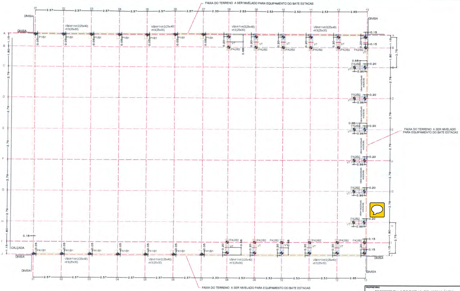
PLANTA BAIXA DE LOCAÇÃO DE ESTACAS escala 1:50
