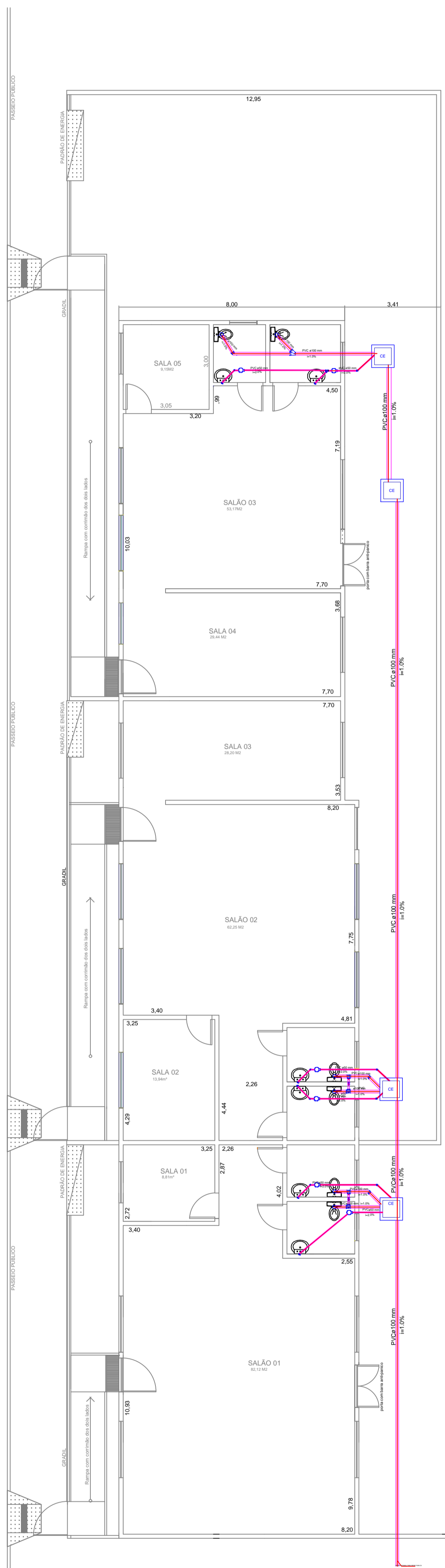
PLANTA BAIXA REDE DE ESGOTO ESCALA: 1:100
